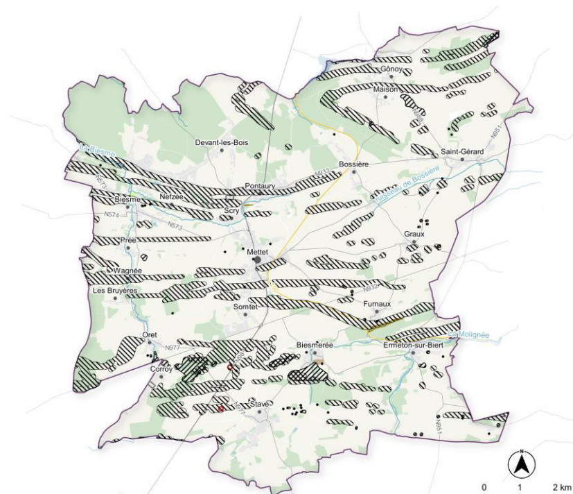
ZONES DGRIM ET ÉBOULEMENT DE VERSANT
